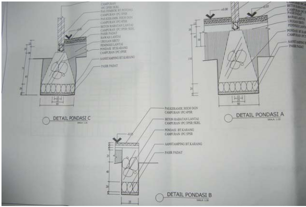
設計図
